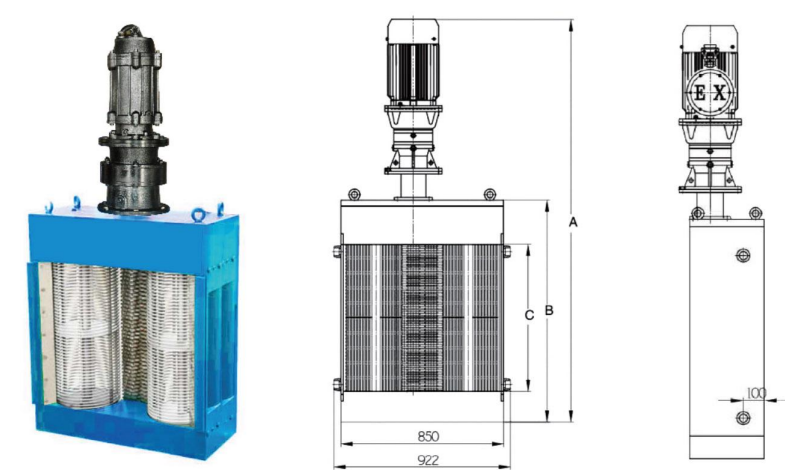
双鼓粉碎型格栅外形图
